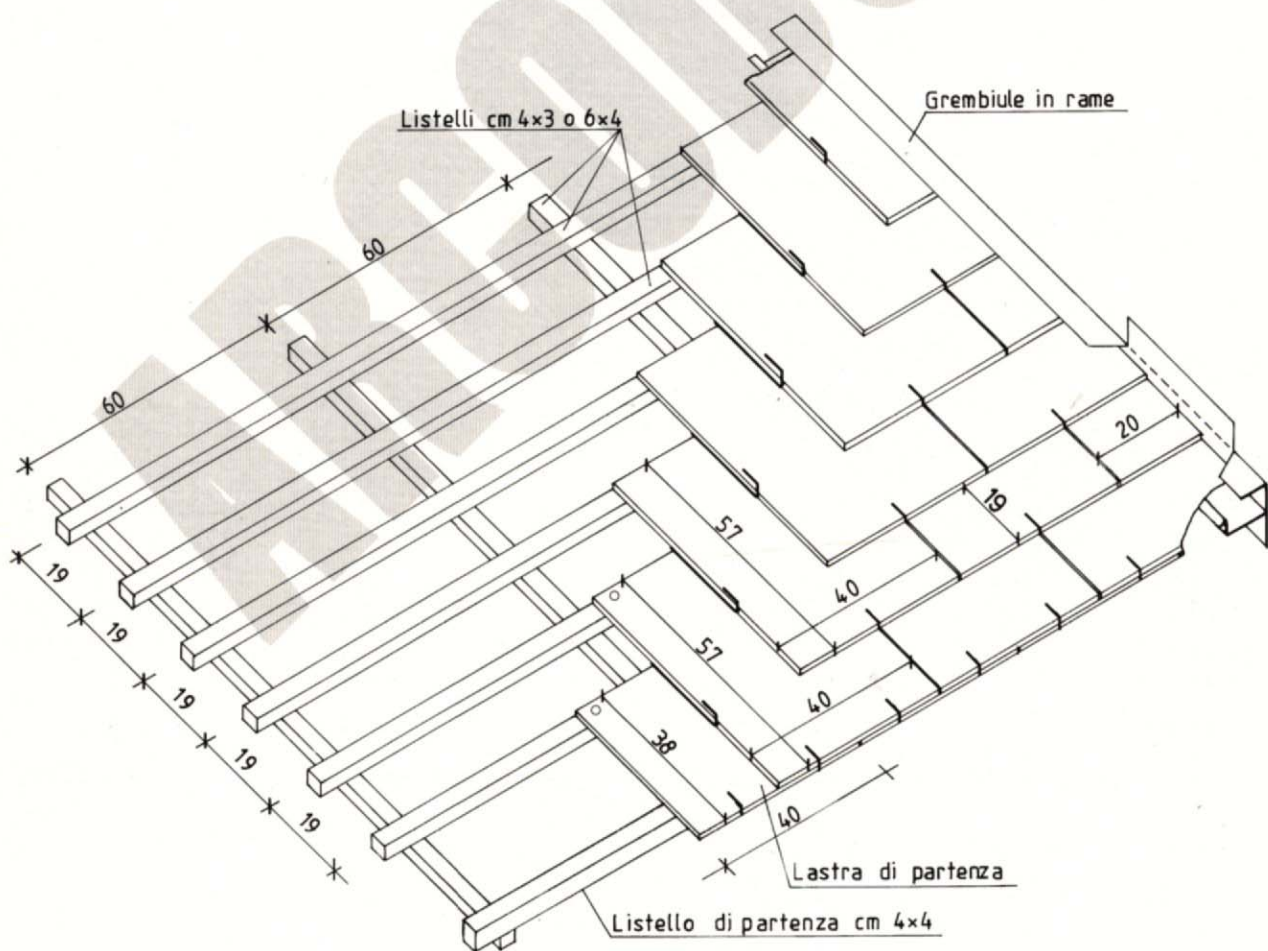
ASSONOMETRIA SCHEMATICA
