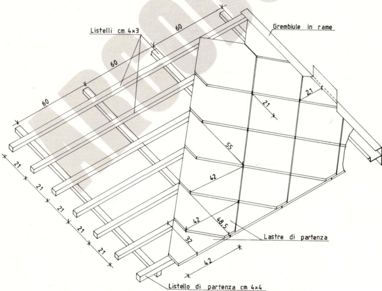
ASSONOMETRIA SCHEMATICA
